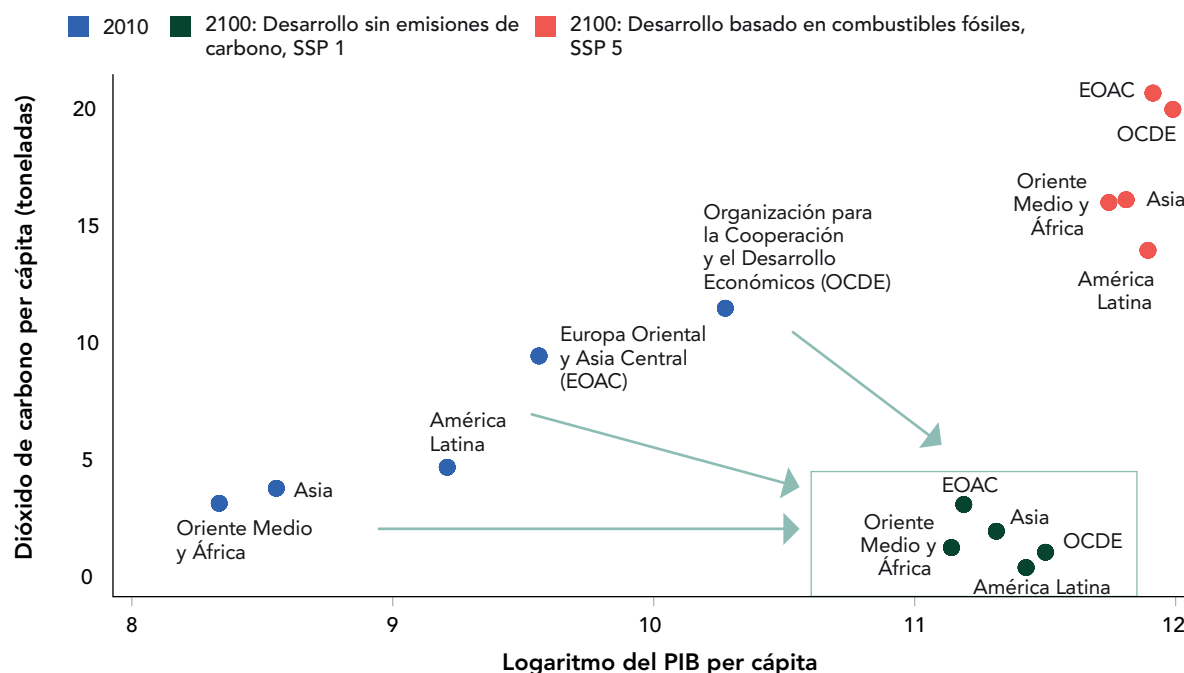
Figura 2. En un escenario de sostenibilidad, para 2100 las regiones disminuyen sus emisiones de dióxido de carbono y aumentan el desarrollo humano
