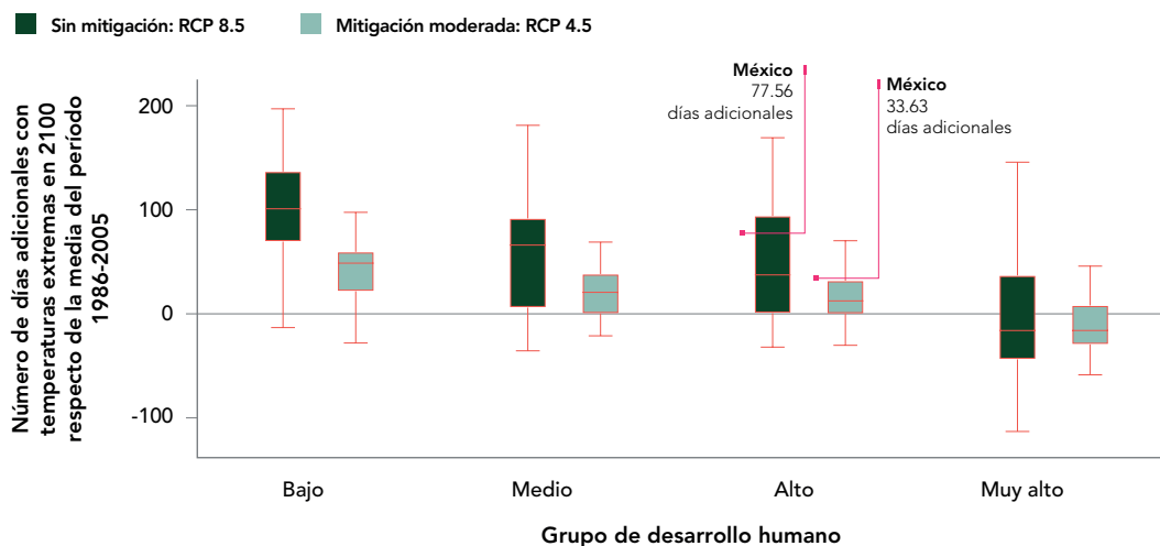
Figura 4. Los cambios en el número de días con temperaturas extremas, como consecuencia del cambio climático, agravarán las desigualdades del desarrollo humano
